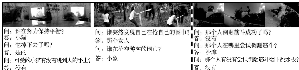
图9-6 视频问答
